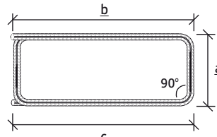
Estribo C5
