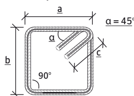
Estribos C1, C6, y E1
