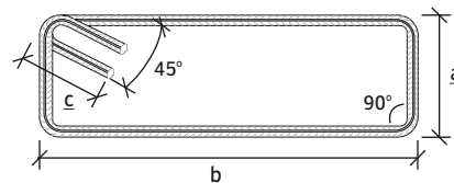
Estribos C2, V1, V2, V3, E2, E3 y E4
